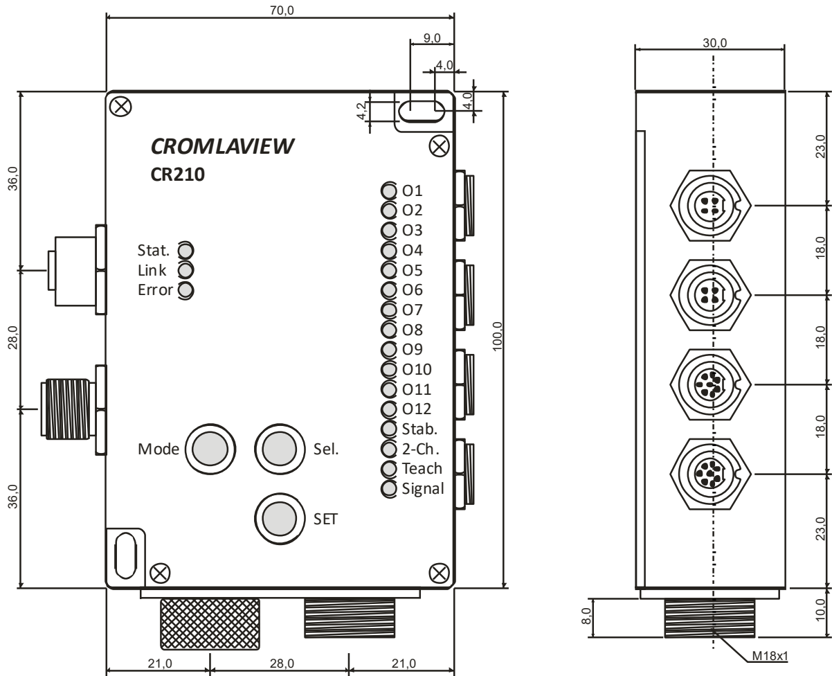
Abbildung 4 : CR210P mit eingebauter Stellvorrichtung für die Driftstabilisierung CROMLASTAB®
