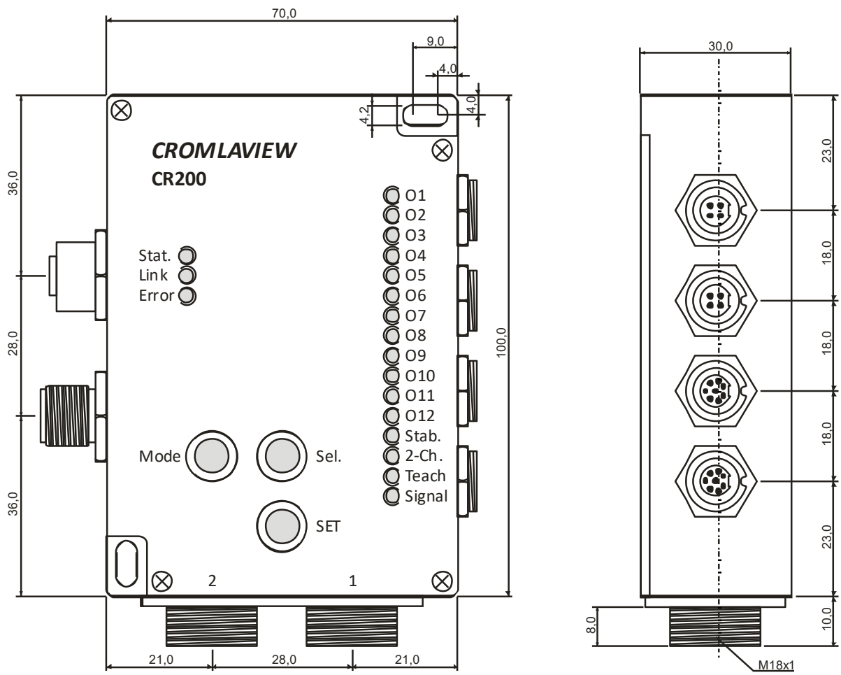
Abbildung 3 : CR200P zum Anschluss von zwei getrennten Lichtleitern
